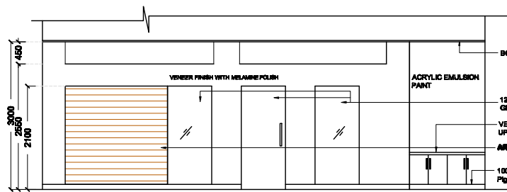
ELEVATION A
