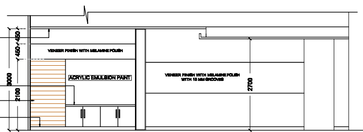
ELEVATION B
