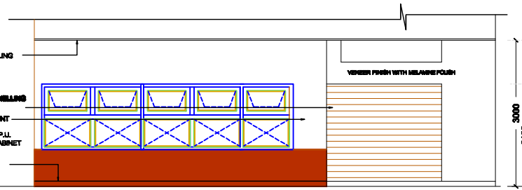
ELEVATION G
